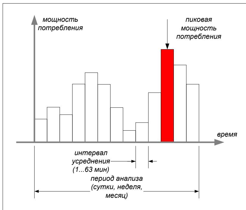
Рис. 11.2 Выбор значения пиковой мощности потребления
