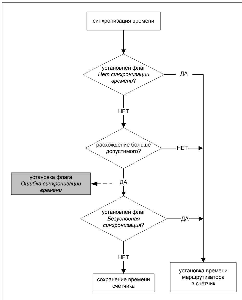
Рис. 8.3 Алгоритм установки флага Ошибка синхронизации времени
