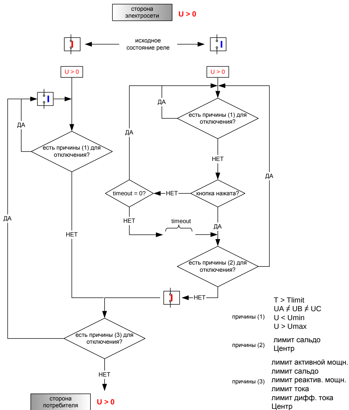
Рис. 5.1 Переподключение счётчика
