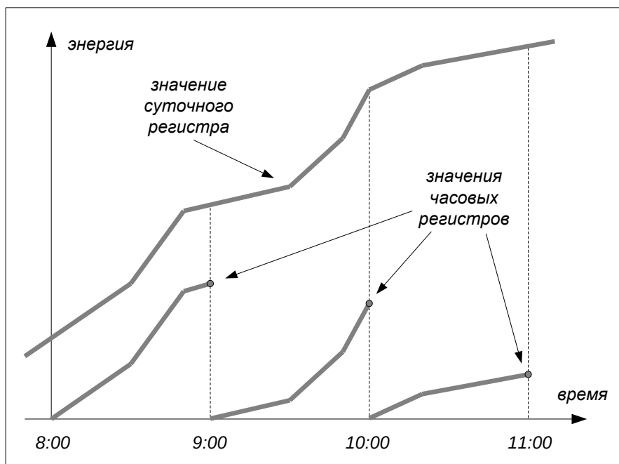
Рис. 10.3 Суточный и часовые регистры (пример)
