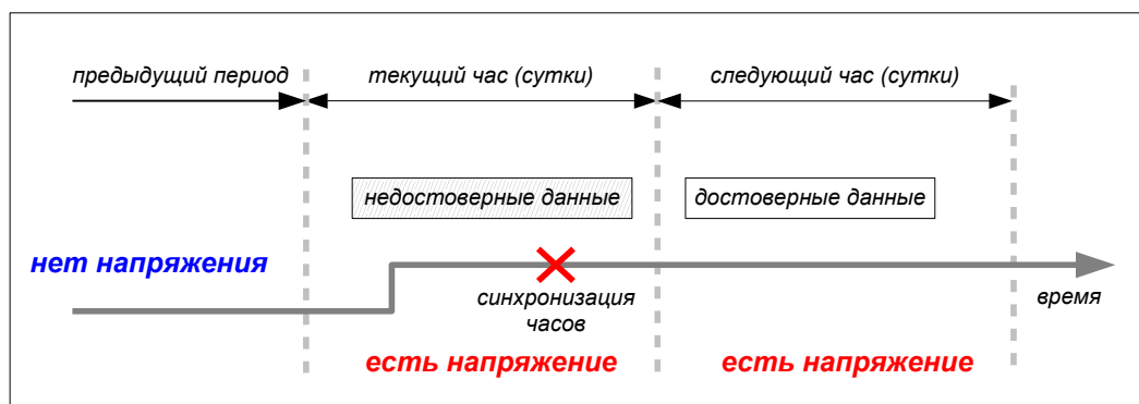
Рис. 8.2 Достоверность данных
